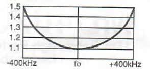
MDC80(3.5MHz)
